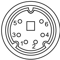
Mini DIN 6-pin (pointing device)
