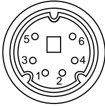
Mini DIN 6-pin (keyboard)
